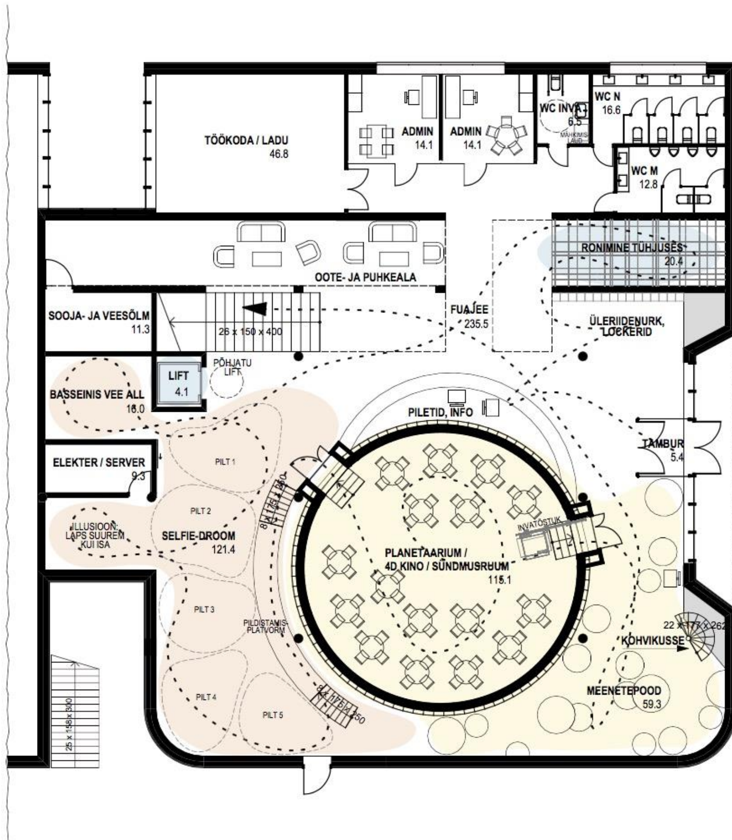
1. KORRUSE PLAAN 1:250
